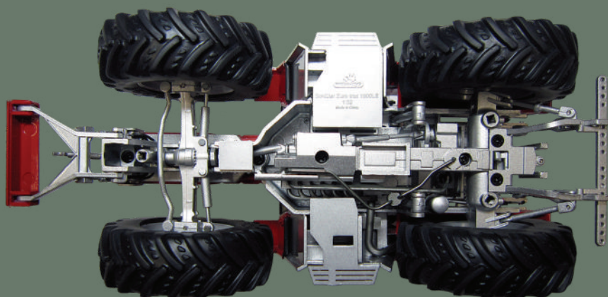
Ansicht von unten mit detailgetreuem Chassis, mit eingesetzter Stoßstange und Ackerschiene.
