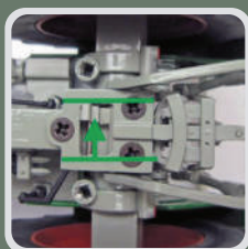
Position 1: Transportposition Verstellhebel an der Unterseite des Modells blockiert die Unterlenker, so dass Anbaugeräte sicher gehalten werden können.
