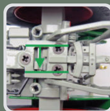
Position 2: Arbeitsposition Verstellhebel an der Unterseite des Modells gibt die Unterlenker frei, so dass Anbaugeräte den Boden erreichen können.
