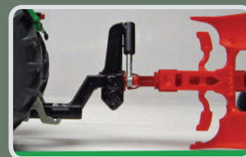
Position 2: Arbeitsposition Verstellhebel an der Unterseite des Modells gibt die Unterlenker frei, so dass Anbaugeräte den Boden erreichen können.
